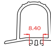
Büyük buzhane kapı lastiği. Great icebox door rubber.
