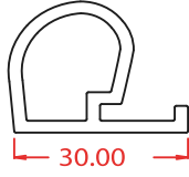
Buzhane kapı lastiği. Ice house doors rubber
