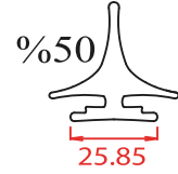
Soğuk oda servis kapı contası. Cold room service door seal.
