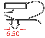
Körüklü mknatıslı conta. Bellows seal magnet
