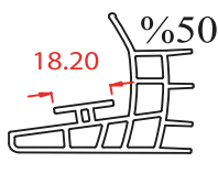
Soğuk oda kapı alt lastiği. Cold room door old tire.
