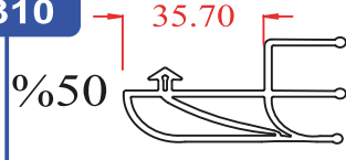
Buzdolabı fitili. Refrigerator wick.
