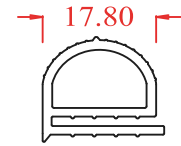
Sanayi tipi buzdolabı kapı fitili Industrial refrigerators door gasket.
